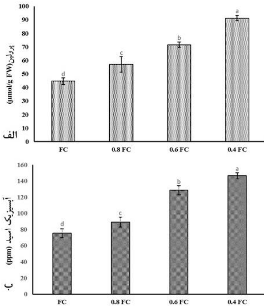
شکل شماره ۱- مقایسه مقدار پرولین (الف) و اسید آسیتزیک (ب) گیاه گلرنگ تحت رژیم‌های مختلف آبیاری، بارهای روی هر ستون بیانگر انحراف معیار می‌باشد.
