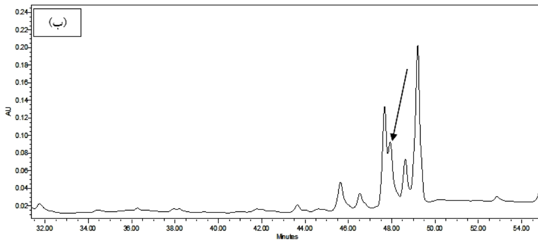
شکل ۴. (الف) کروماتوگرام تاناشینون استاندارد، (ب) کروماتوگرام تاناشینون ریشه در تیمار تغذیه خاکی با ۱۰۰۰ ppm نانو اکسید سریم در مرحله زایشی.
